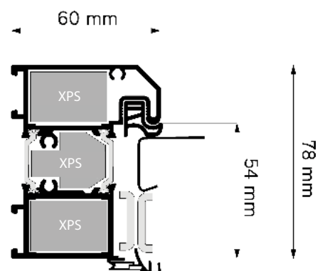
Aluthermo frame
