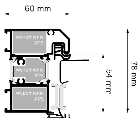
Ościeżnica Aluthermo 73
